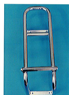
Bad- och räddningsstege , rostfri. Ø 25 mm. Bredd 18 cm. Materialtjocklek 1,5 mm. Längd nedfäld 70 cm, uppfäld 50 cm.
