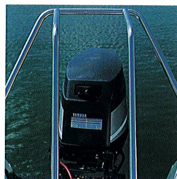
"Snobbåge" , en praktisk akterpulpit, som ger bra greppmöjligheter runtom motorbrunnen. Finns i två bredder. Ø 25 mm. Materialtjocklek 1,5 mm.
