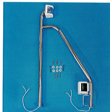
Rostfri stävpulpit med sido- och topp-lanterna, komplett med kabel. Ø 25 mm. Materialtjocklek 1,5 mm.
