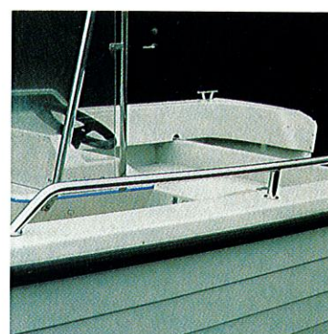
Rostfritt grabbräcke. Levereras i par. Längd 170 cm. Höjd 10 cm. Ø 25 mm. Materialtjocklek 1,5 mm.
